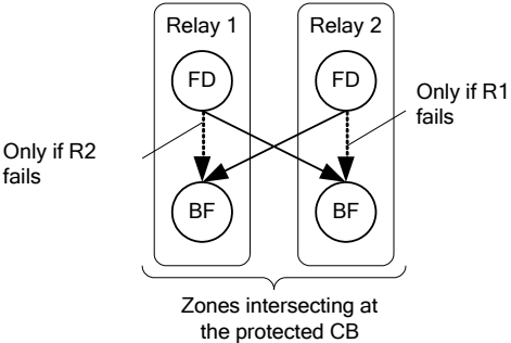
(d) Cross-check scheme w/ switchover
